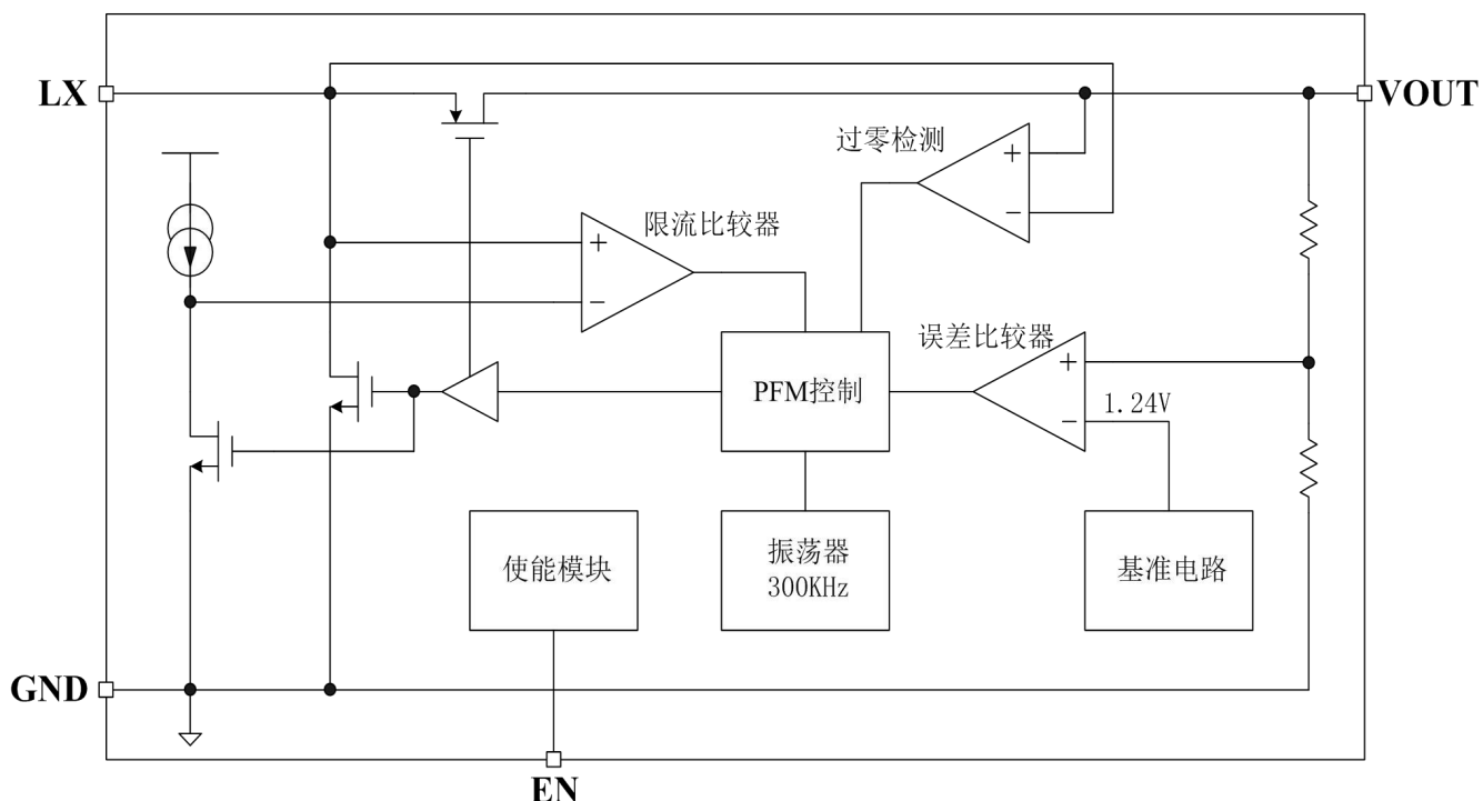
图 2: HX2304 的内部电路方框图
