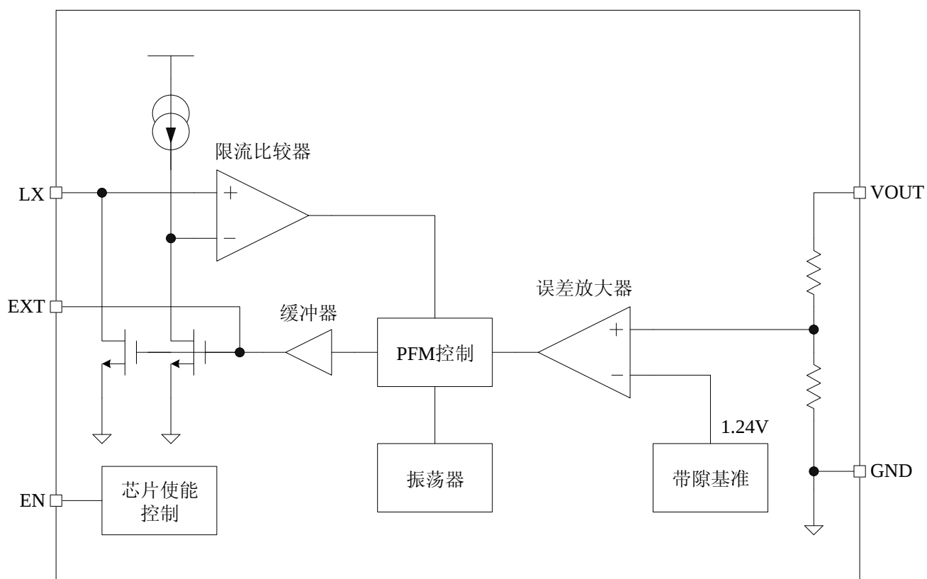
图 2: HX2303 的内部电路方框图
